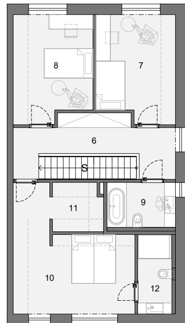
OBJEKT A5 byt A _ PŮDORYS 2.NP
